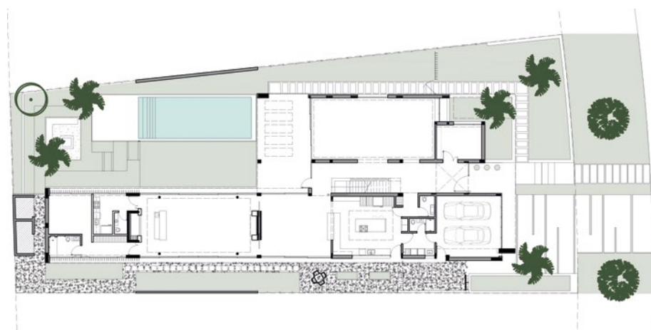
PLANTA BAJA
