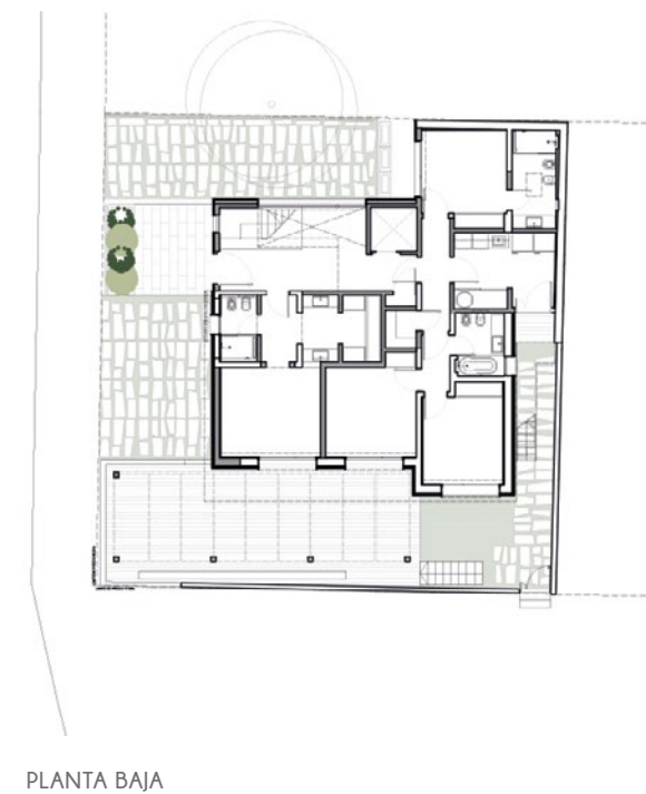
PLANTA BAJA
