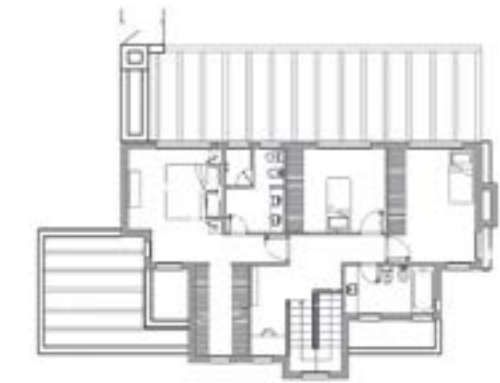
PLANTA ALTA
