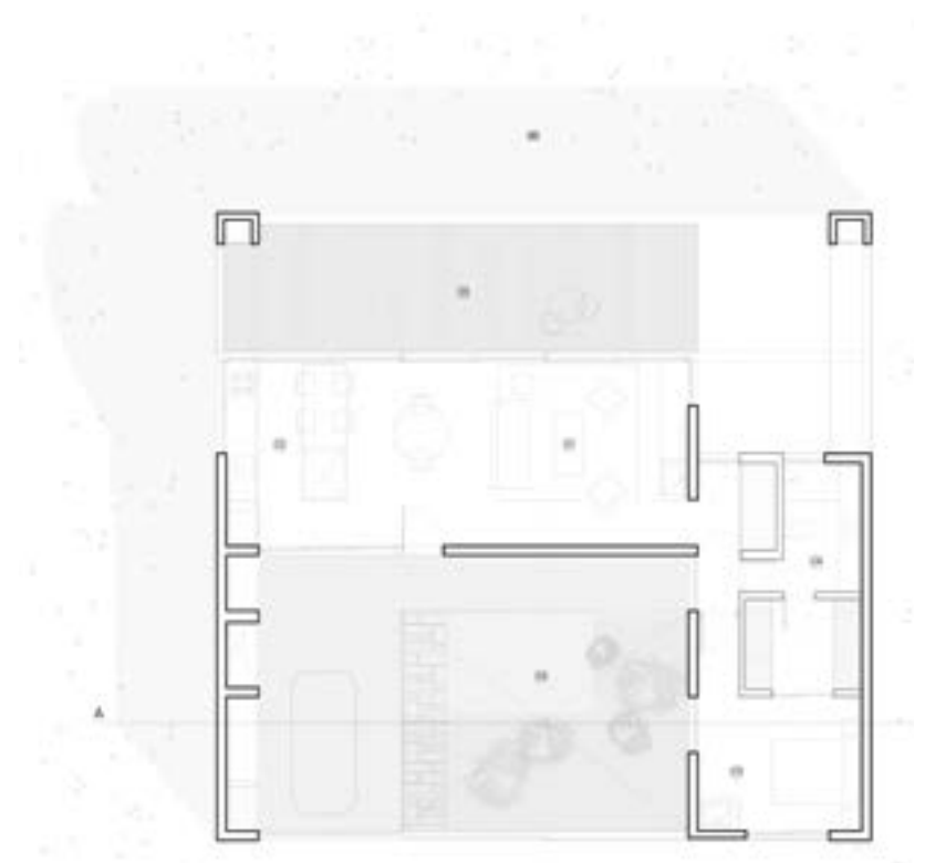
PLANTA
