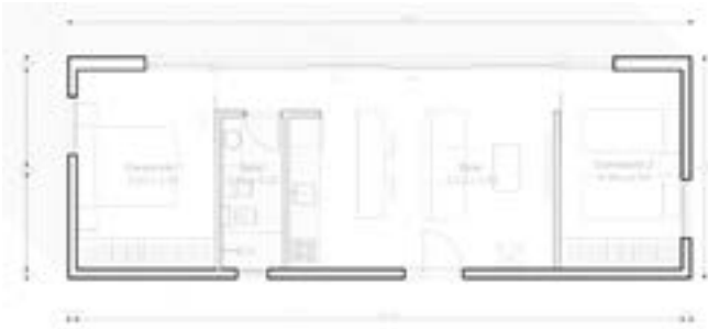
PLANTA 2 DORMITORIOS
